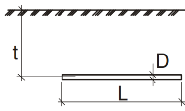
Рис.1.4. Расчетные схемы расположения горизонтального заземлителя
